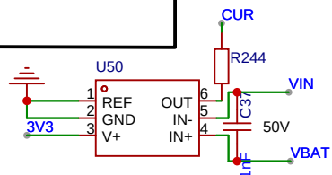
电流计
