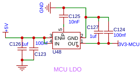
MCU LDO
